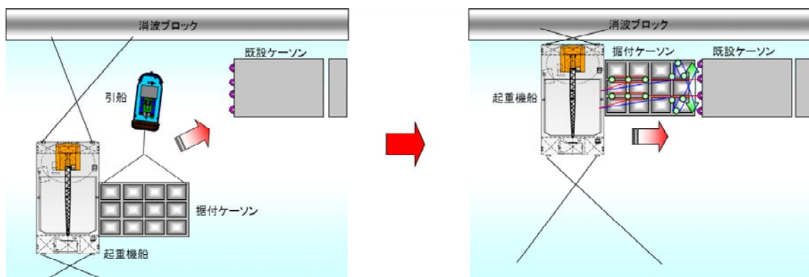
【ケーソン据付状況図】
