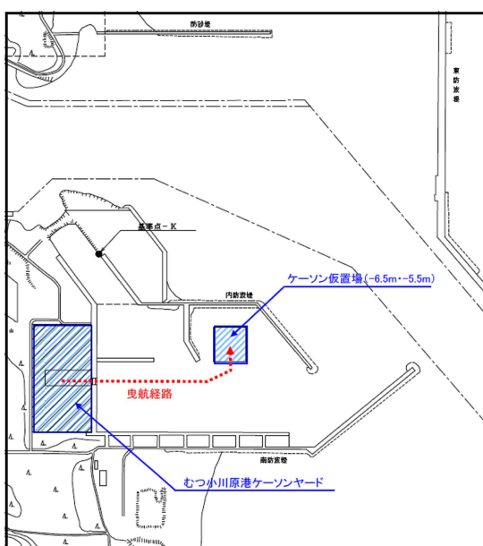
【施工位置図】
