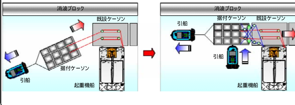
【ケーソン据付イメージ図】
