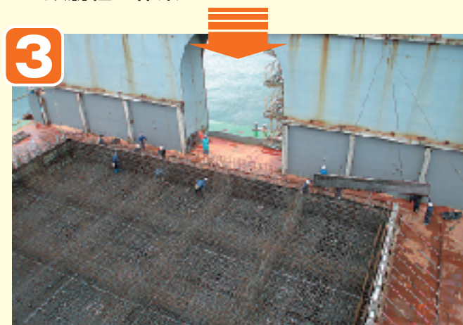
●型枠組立作業
