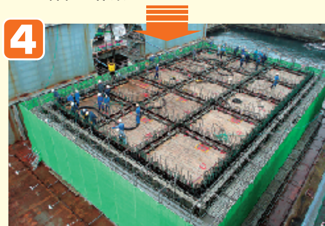
●コンクリート打設作業
