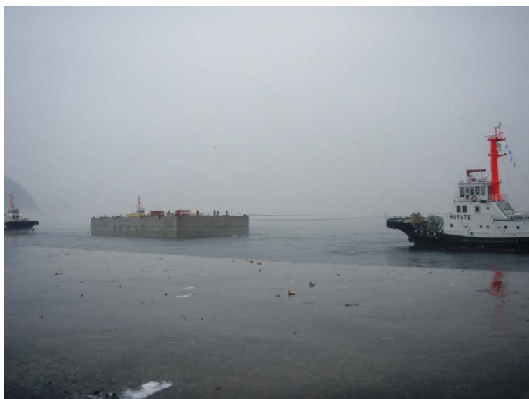
▲ケーソン曳航状況
