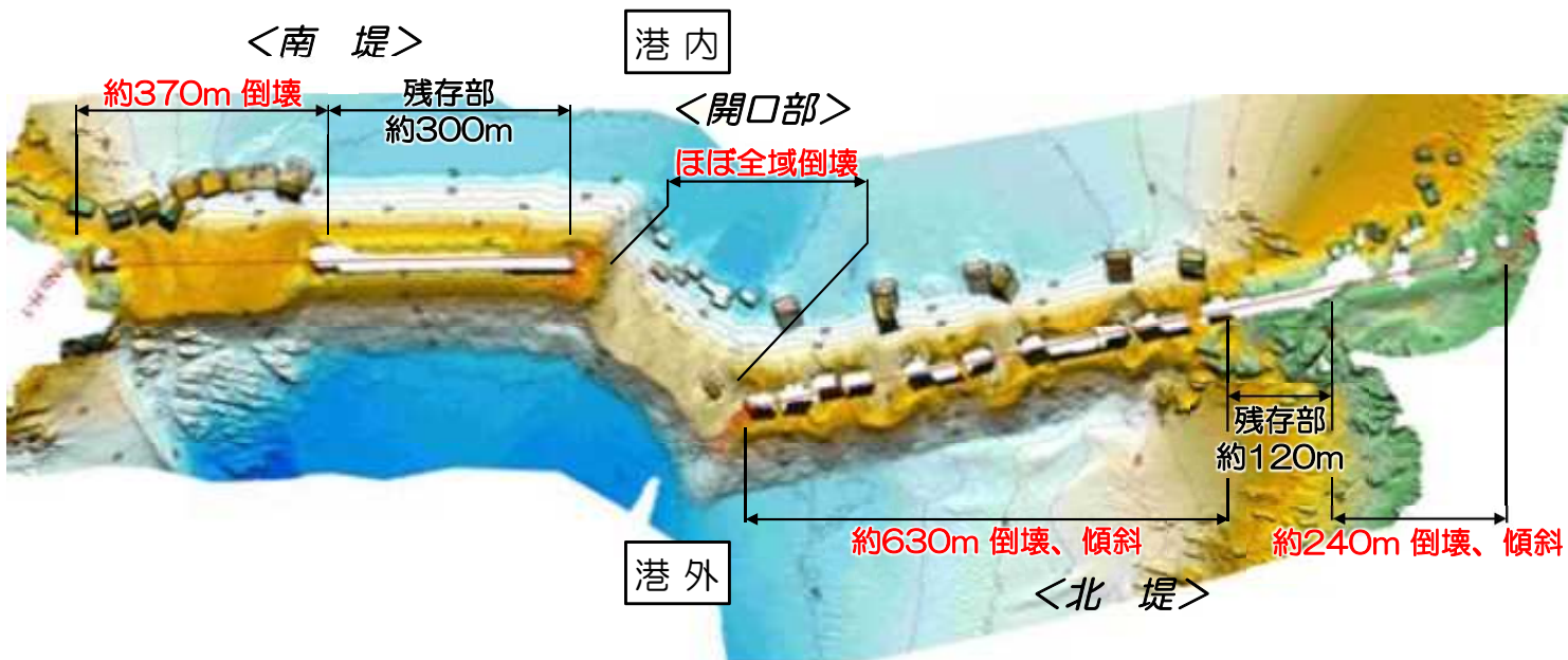
マルチビーム測量結果（面的に海底を測量した結果）
