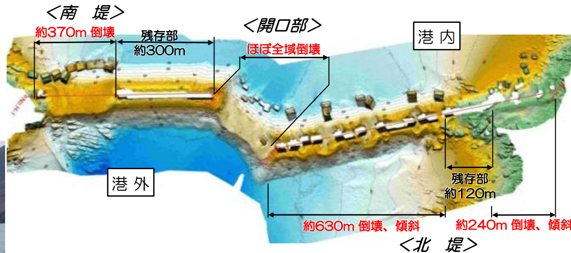
ナローマルチビーム測量結果 (面的に海底を測量した結果)
