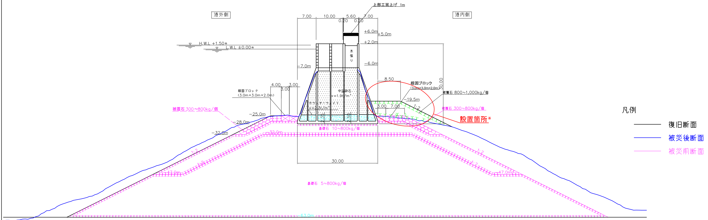
湾口防波堤（南）（深部）4区標準断面図
