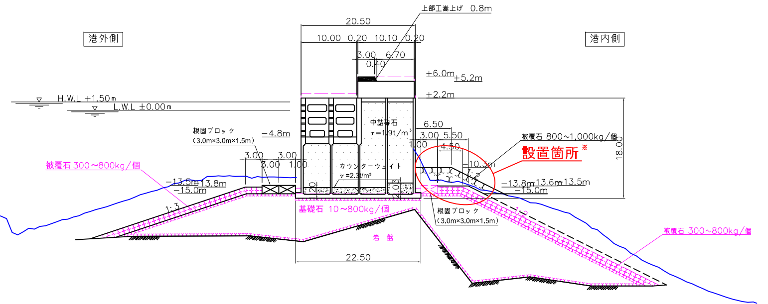
湾口防波堤（南）（深部）4区標準断面図
