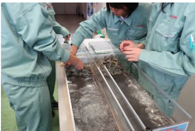
波消しブロックの効果を模型で実験
