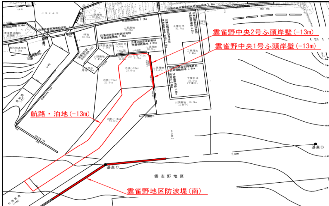
石巻港 災害復旧対象施設位置図(国施工分)
