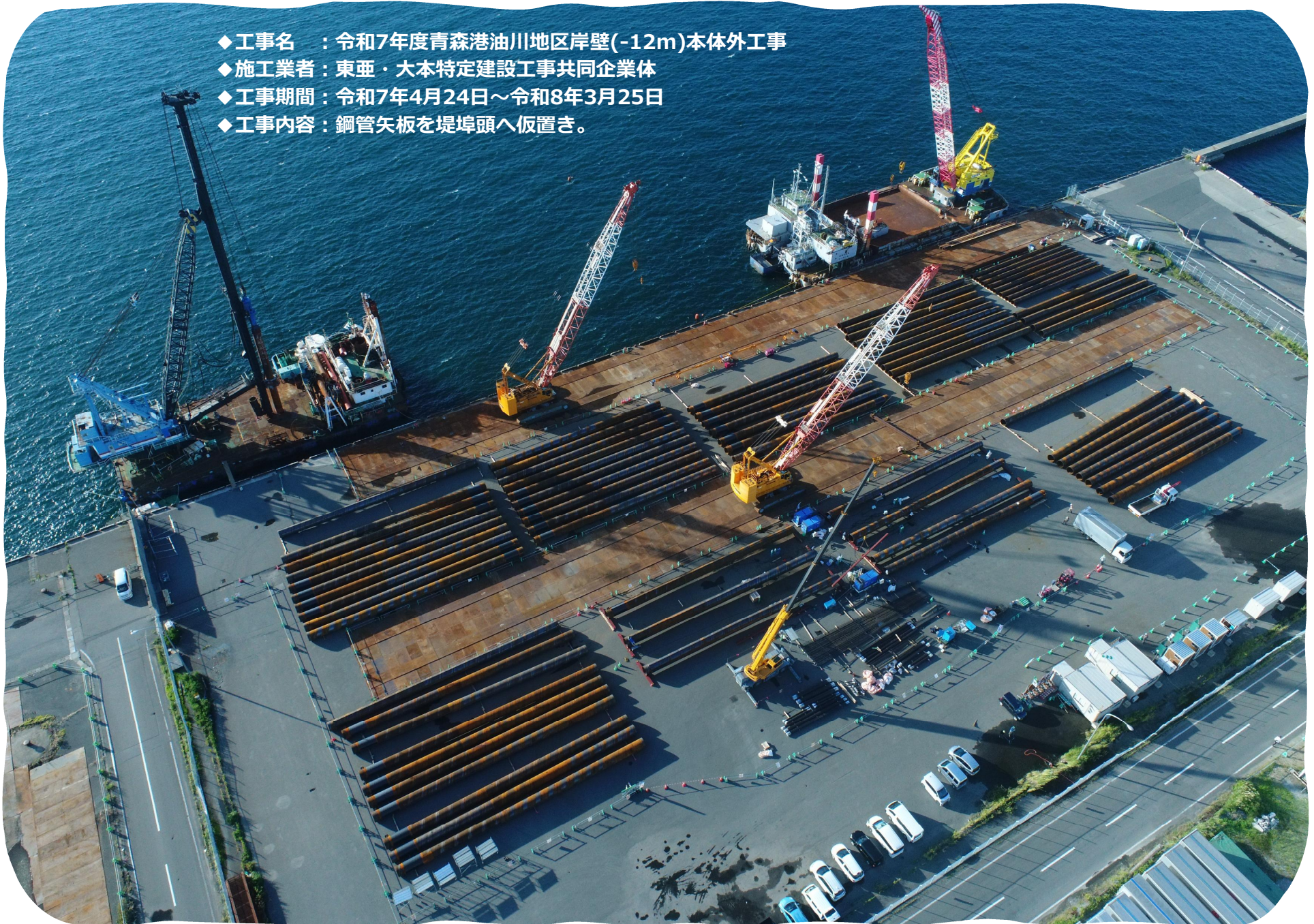
鋼管矢板仮置き
