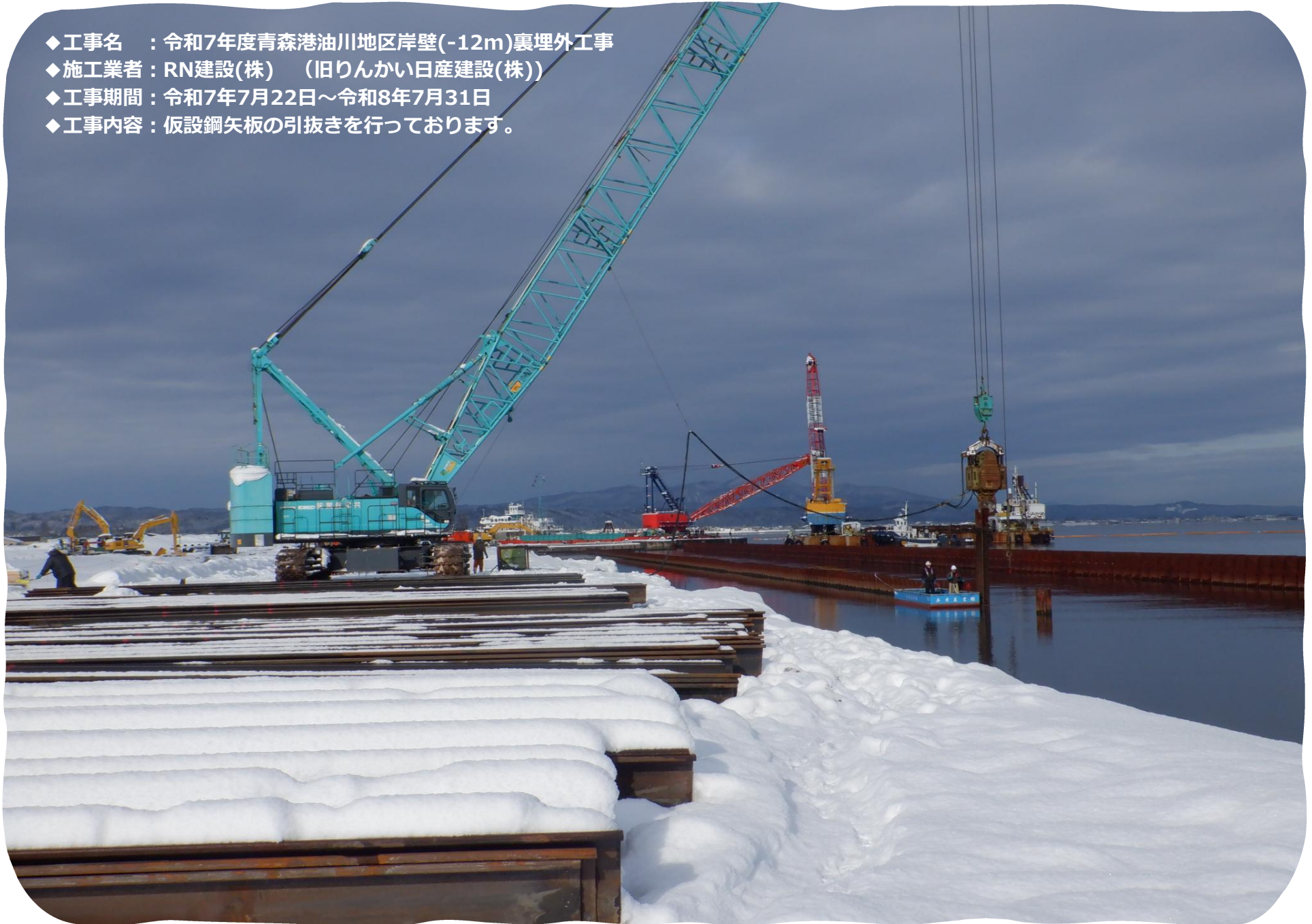
仮設鋼矢板の引抜き
