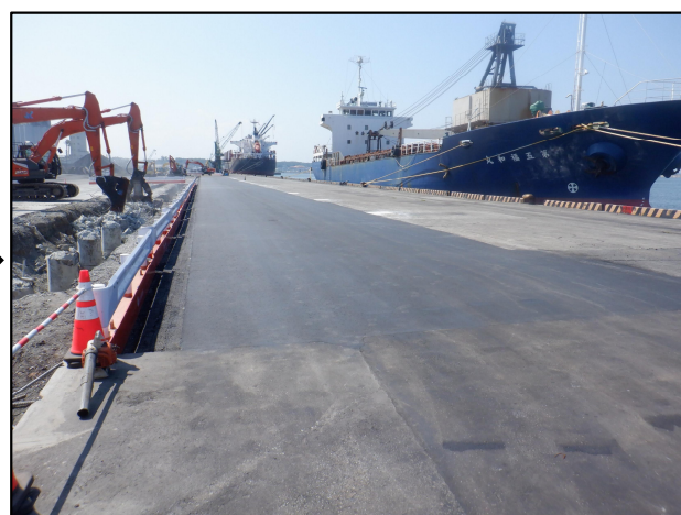
R8.8.6新設アスファルト舗装施工完了
