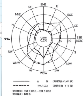
風向風速図
