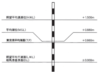
潮位図
