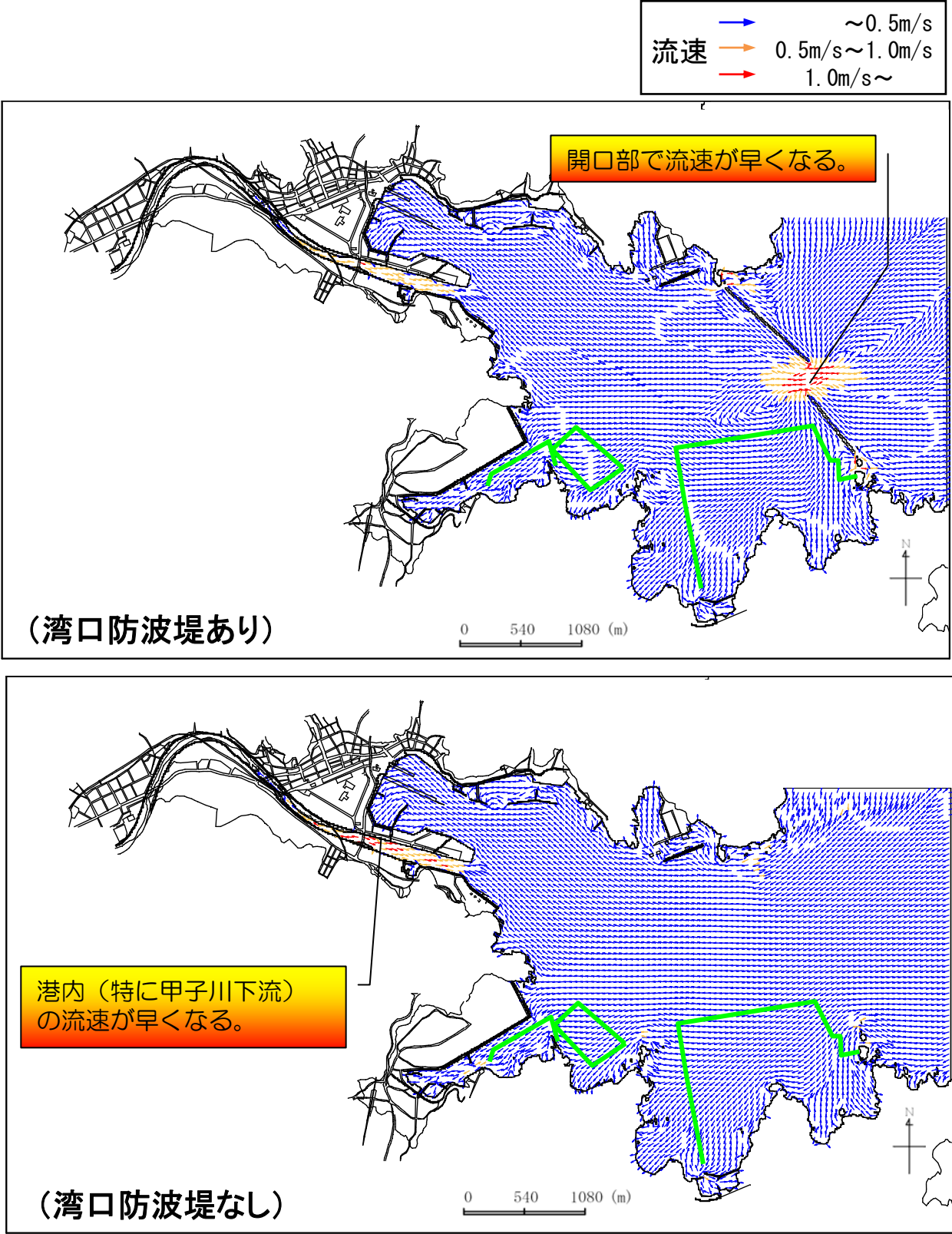
▼図 釜石港の湾口防波堤あり、なしの地形における2010年チリ地震津波の流速分布
