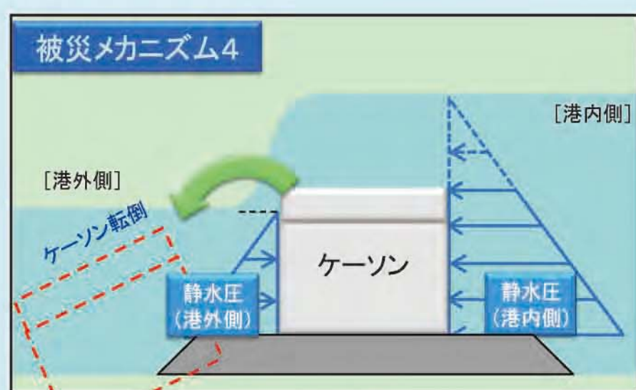
引き波
