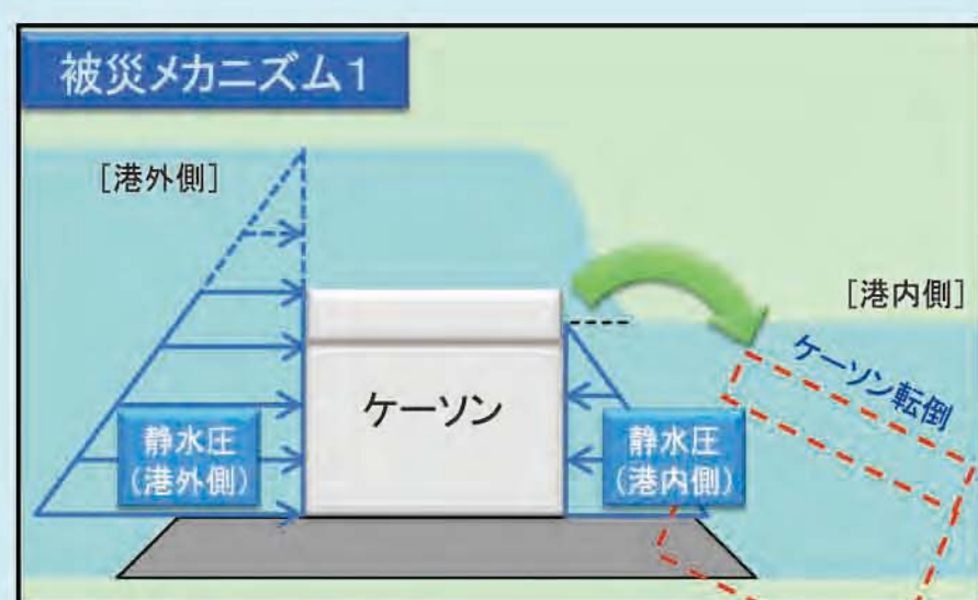
押し波
