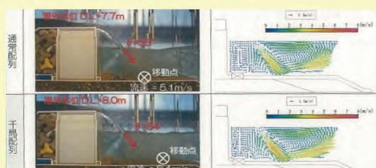
模型実験
