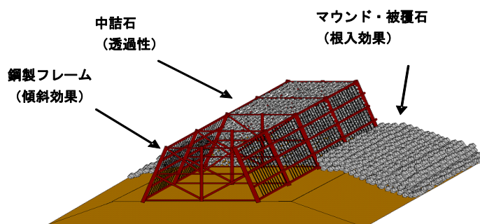
図-1 鋼製フレーム工法のイメージ図
