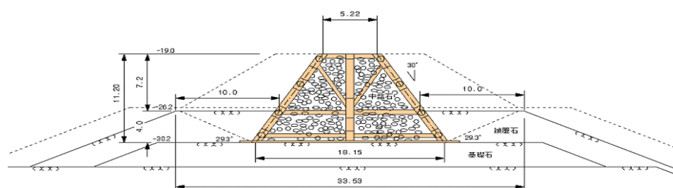
図-2 鋼製フレーム工法の試設計例 (台形根入式潜堤)
