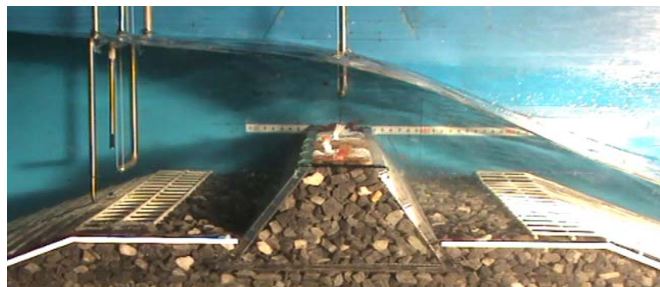
図-3 水理実験状況
