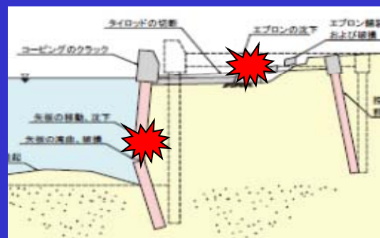
矢板岸壁
