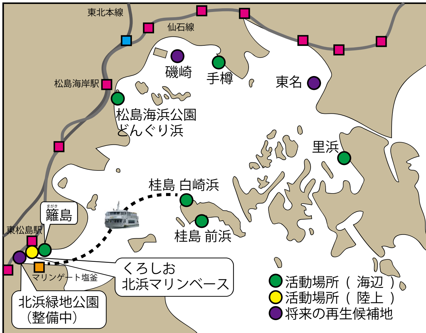
まつしまわん 松島湾のアマモ場再生の活動MAP
