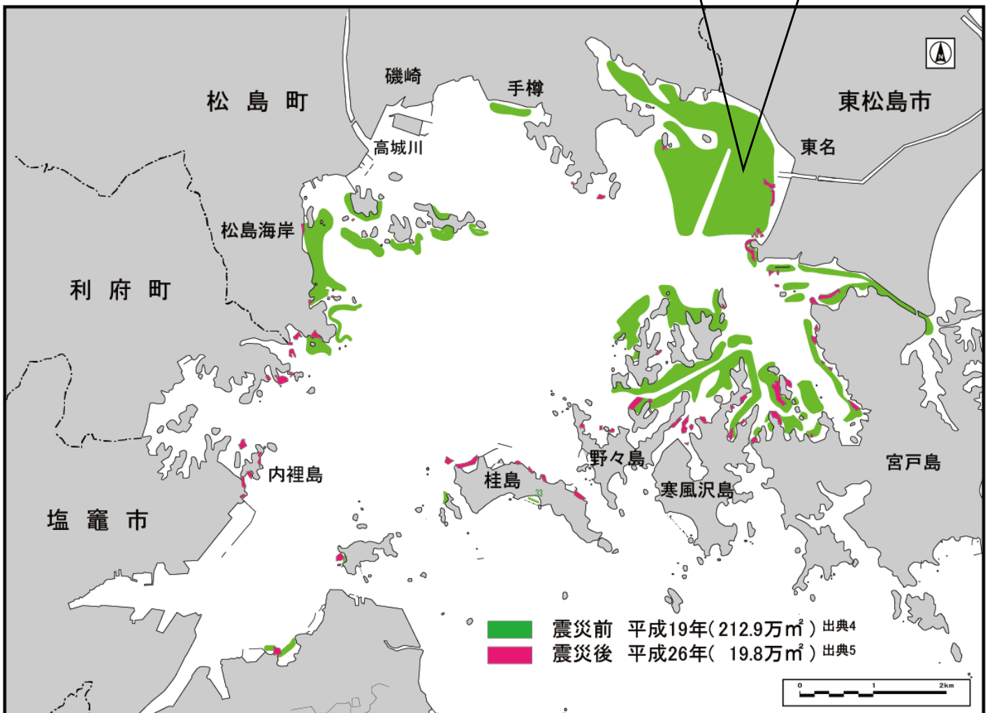
震災前と震災後のアマモ場
