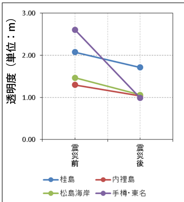
震災前と震災後の海水の透明度
