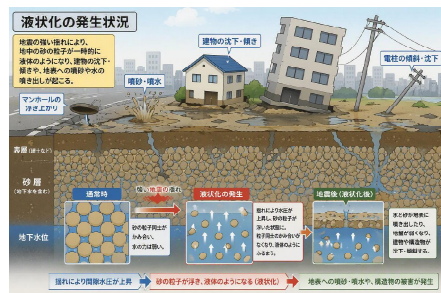
地盤の液状化現象
